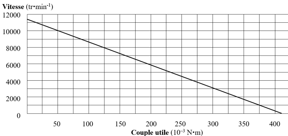
Courbes caractéristiques du moteur : Vitesse = f(couple)
