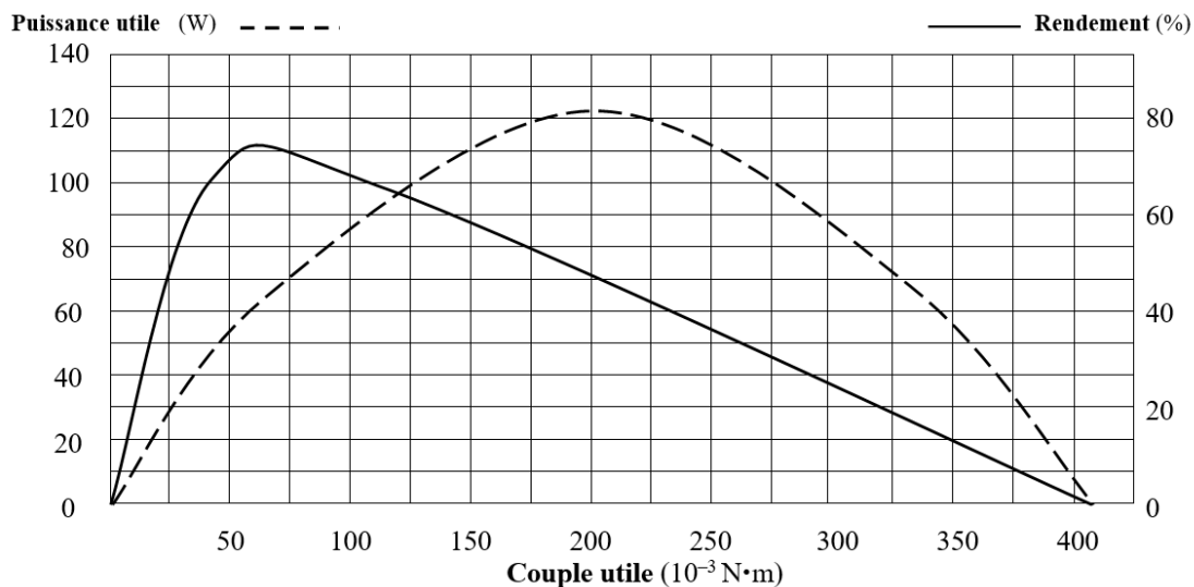
Courbes caractéristiques du moteur : Puissance utile = f(couple) Rendement = f(couple)
