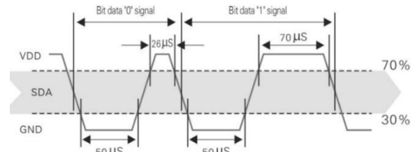
Figure 7 : détails des états 0 et 1 des bits
