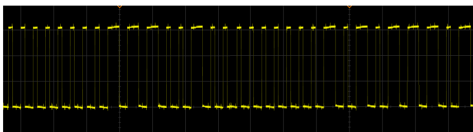
Figure 5 : trame à compléter par les bits de parité
