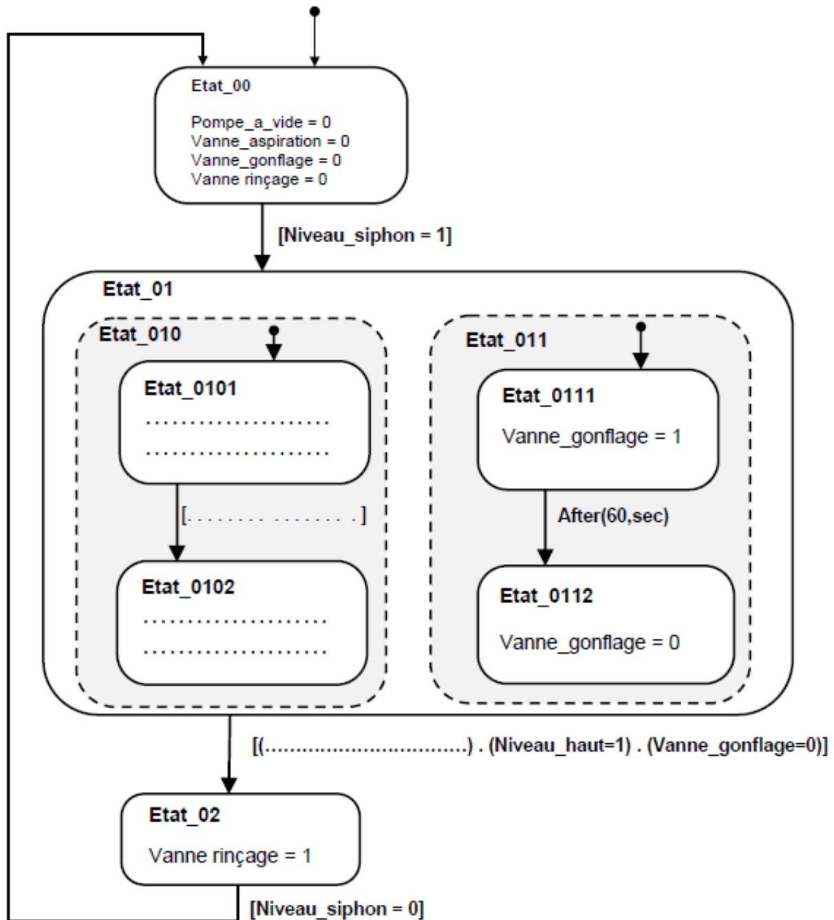
Diagramme d'état de la fonction rincer
