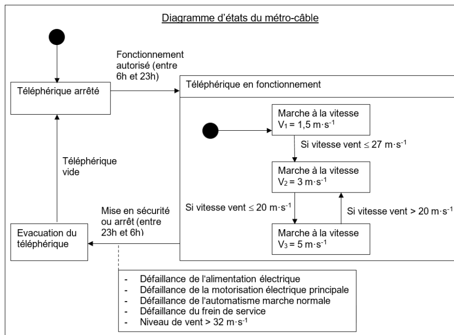
Figure 2 : diagramme d'états du métro-câble
