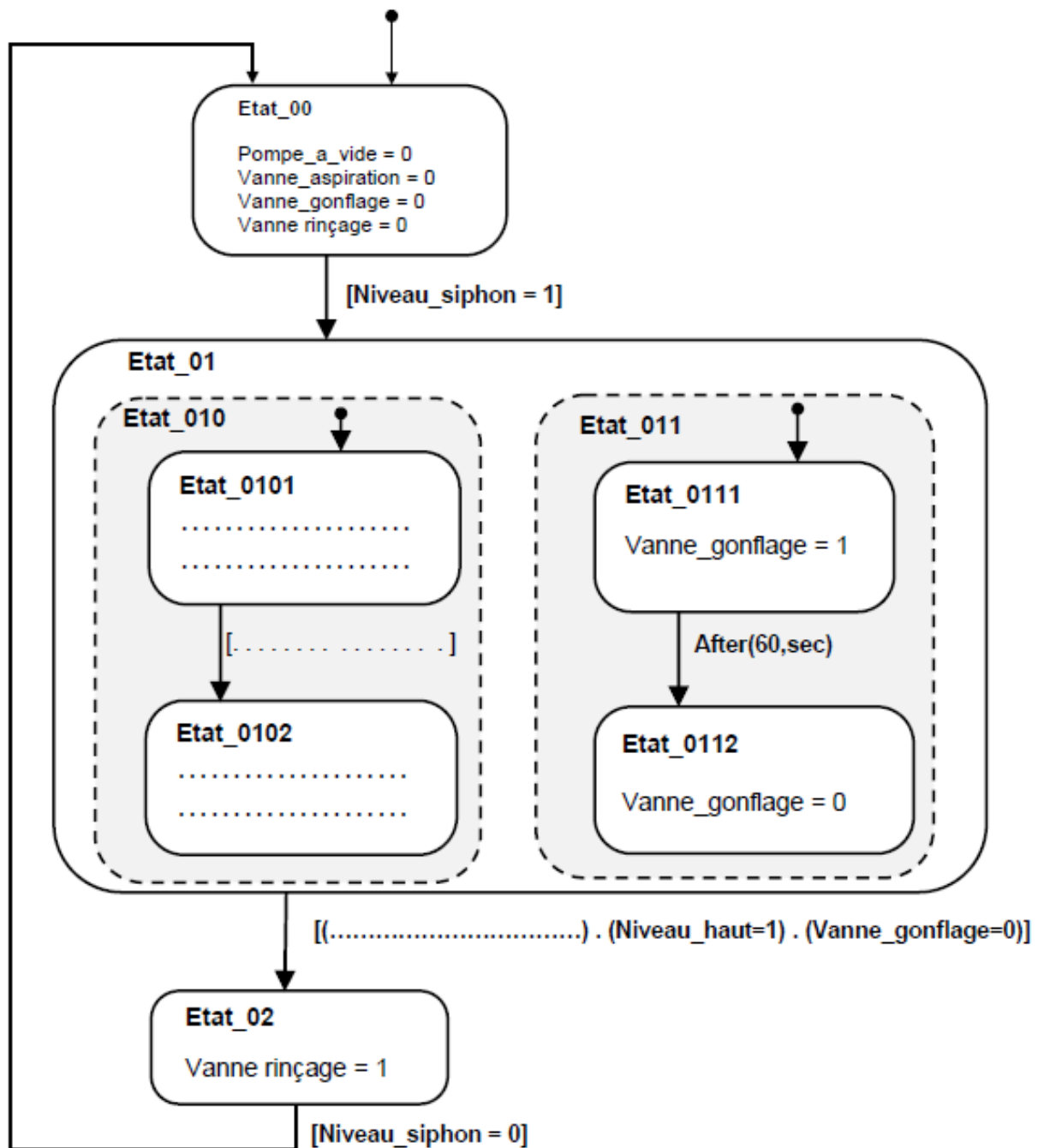
Diagramme d'état de la fonction rincer
