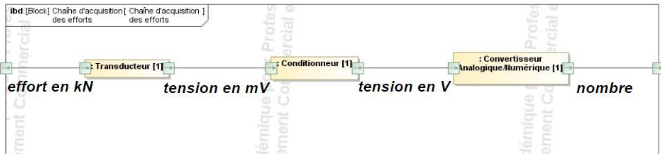
Figure 2 : chaîne d'acquisition de l'effort dans le hauban 17
